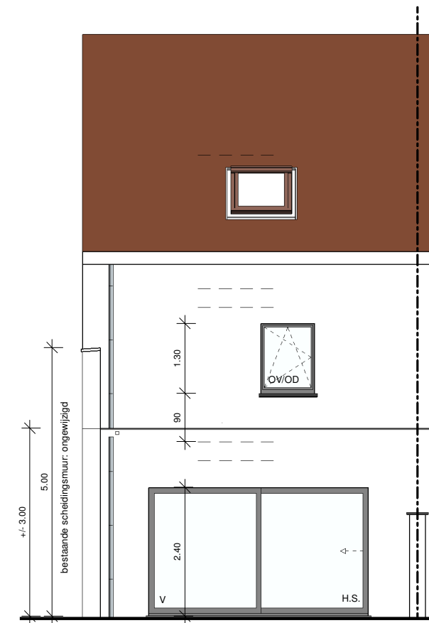
2 Achtergevel - Woning 4
