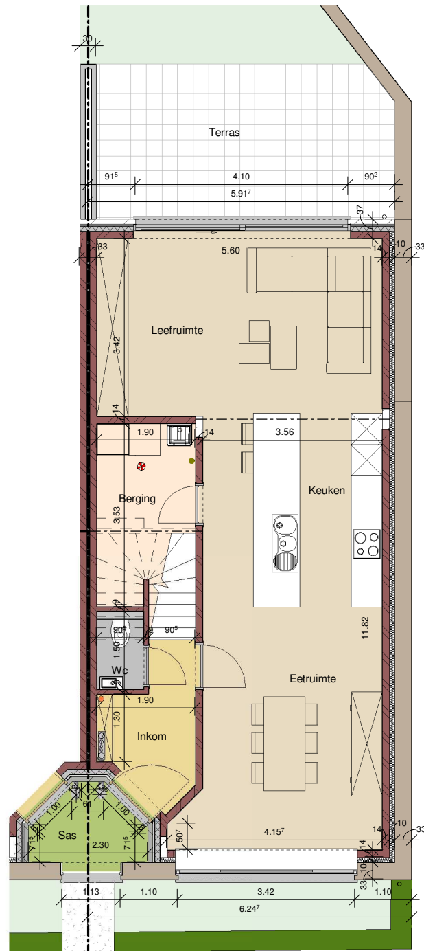
1 Gelijkvloers - Woning 4
