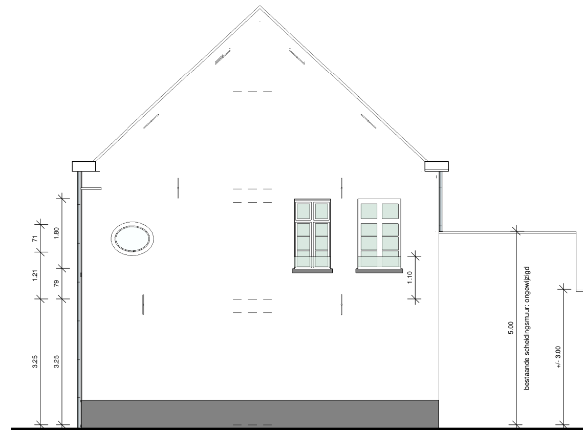
3 Zijgevel - Woning 4
