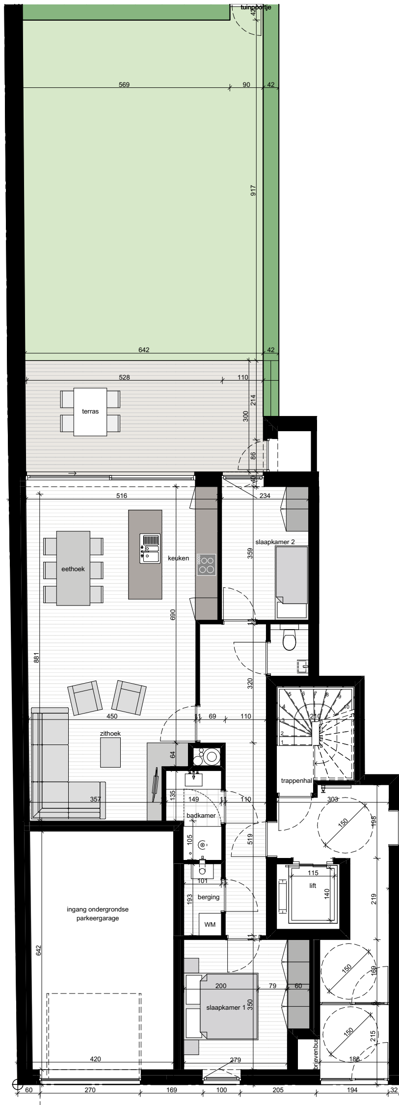
APPARTEMENT 0.1
