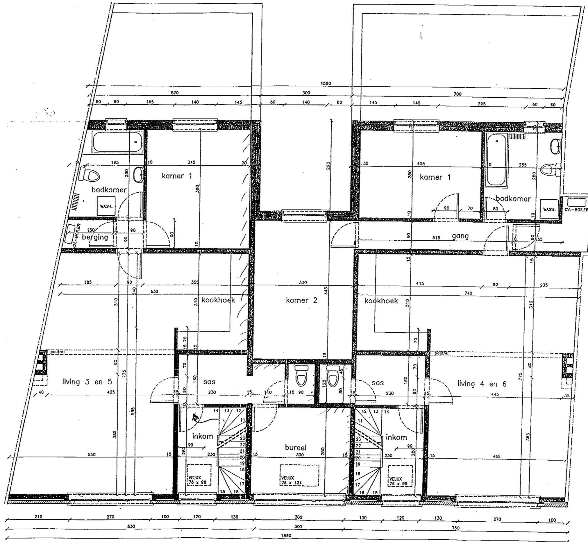
Plan verdieping 1 en 2
