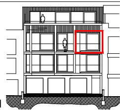
Zuidgevel
